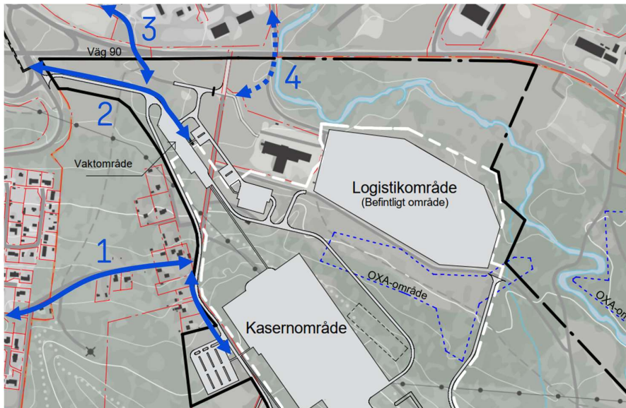
Figur 3-1. Rekommenderade gång- och cykelanslutningar (1–3). Alternativ 4 avskrivs.
