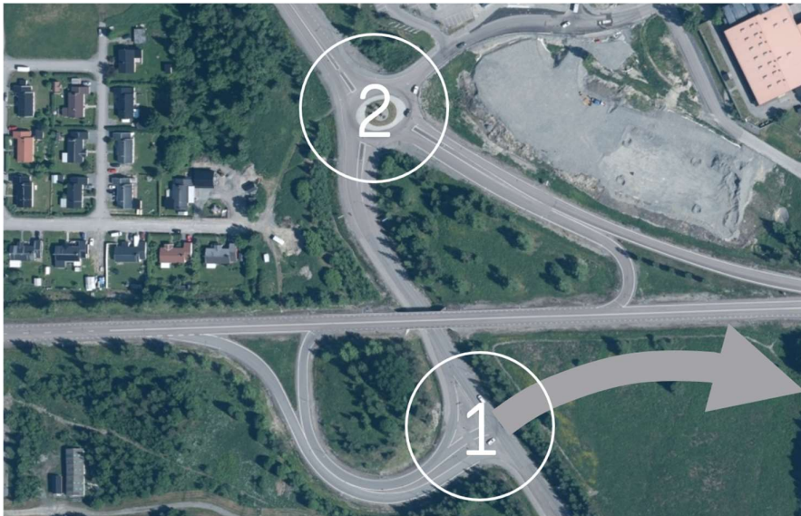
Figur 4-2. Enligt Swecos förslag ansluts regementet till det allmänna vägnätet i den södra delen av trafikplats Hågesta (korsning 1). Bildkälla: Lantmäteriet, redigerad av Sweco.
