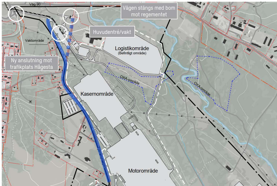
Figur 3-2. Förslag på vägnät och utformning av regementsområdet. Blå heldragen markering visar Tjärnmyrvägens framtida och delvis förändrade vägsträckning. Blå streckad markering visar befintlig vägsträcka som tas bort.
