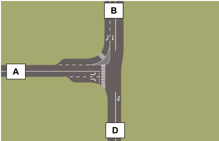
Figur 4-3. Korsningens schematiska utformning i Capcal, nuläge. A avser väg 90, B avser Söderleden norrut och D avser Söderleden söderut.
