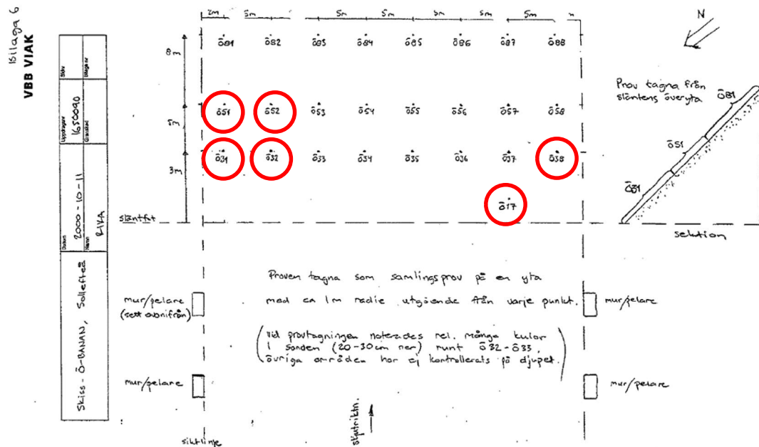
Figur 6 Utdrag från VBB VIAK AB:s sjätte bilaga. Skissen visar punkternas placering i kulfångnet. Röda cirklar visar de områden där blyhalter över riktvärdet för MKM påträffades.
