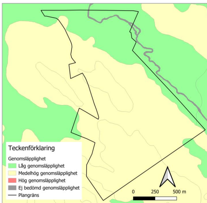
Figur 3-3. Genomsläpplighet i utredningsområdet och dess omgivning (källa: SGU:s digitala kartverktyg).
