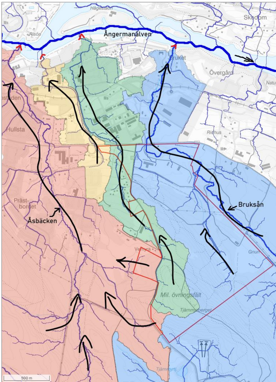
Figur 3-5. Befintliga avrinningsområden och ytliga flödesvägar (blå linje) inom planområdet (röd linje) med omnejd. Bakgrundskarta: Lantmäteriet (SCALGO Live).
