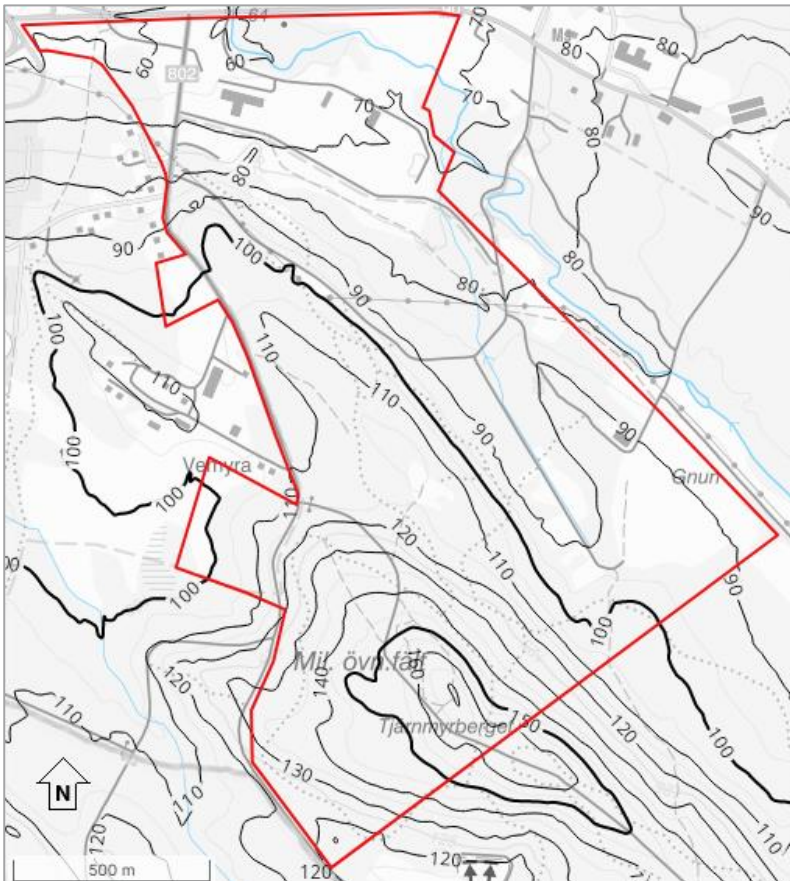
Figur 3-4. Höjdkarta med konturlinjer (5 m). Höjddata: Lantmäteriet. (SCALGO Live).
