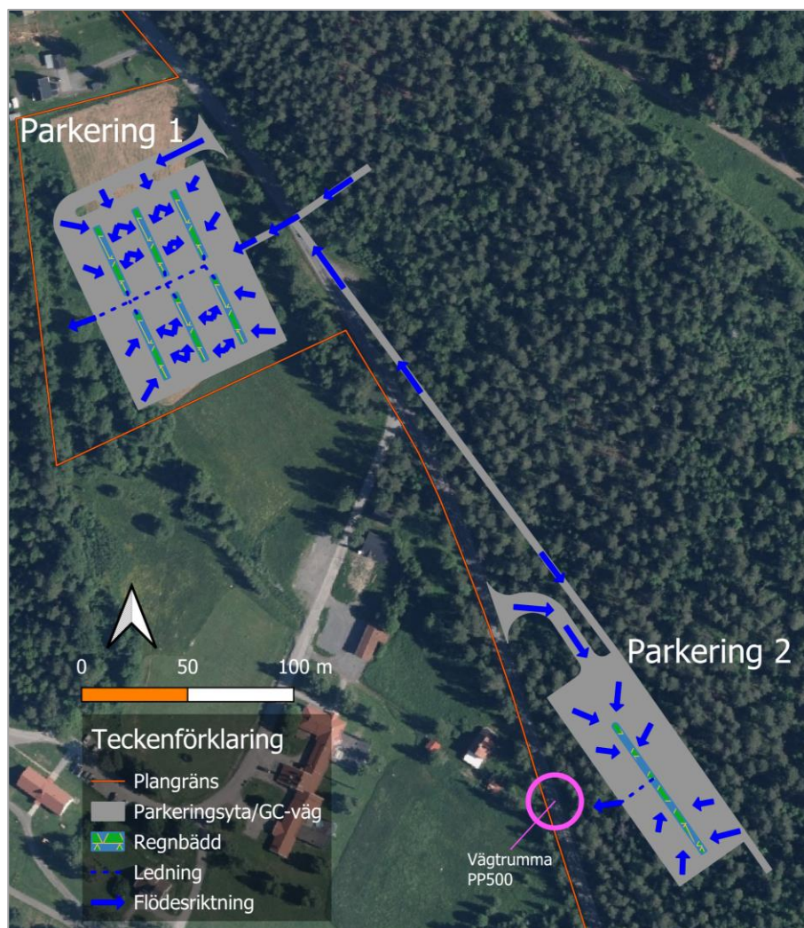
Figur 8-3. Principskiss över förslag på placering av anläggning för fördröjning av dagvatten, med pilar som visar föreslagna rinnvägar.
